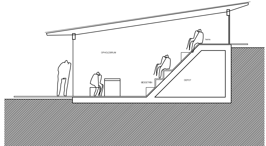
Snit 1:100
